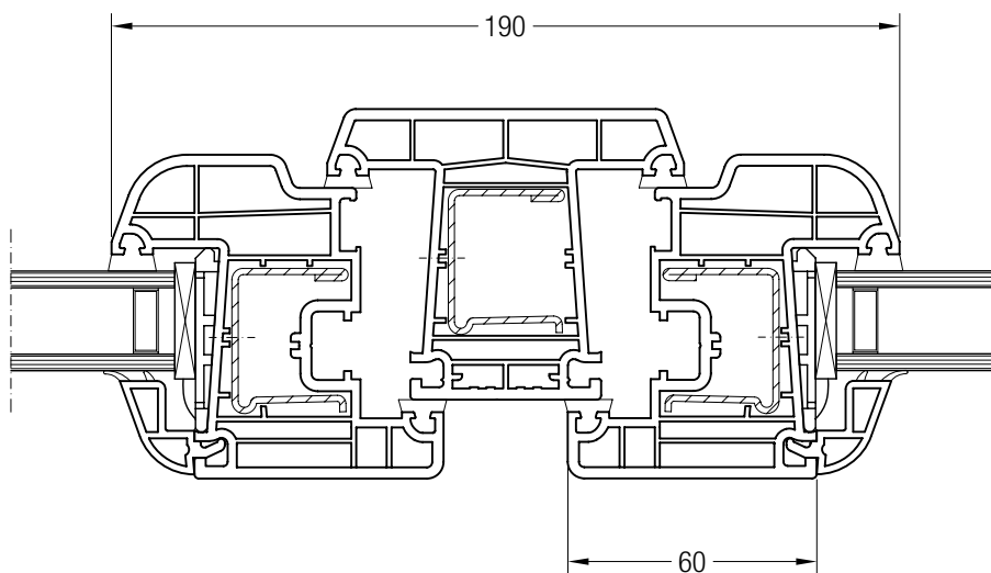
Pfosten 86 ED70 mit Flügel 60 rund ED70, 1550460
