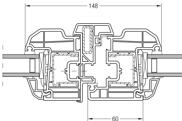
Stulpprofil Bautiefe 70 mit Flügel A 60 ED70, 1550051
