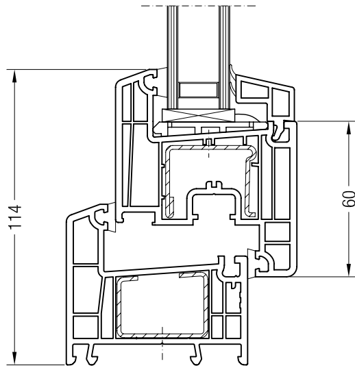
Blendrahmen 62 ED70 mit Flügel Z 60 ED70, 1550413
