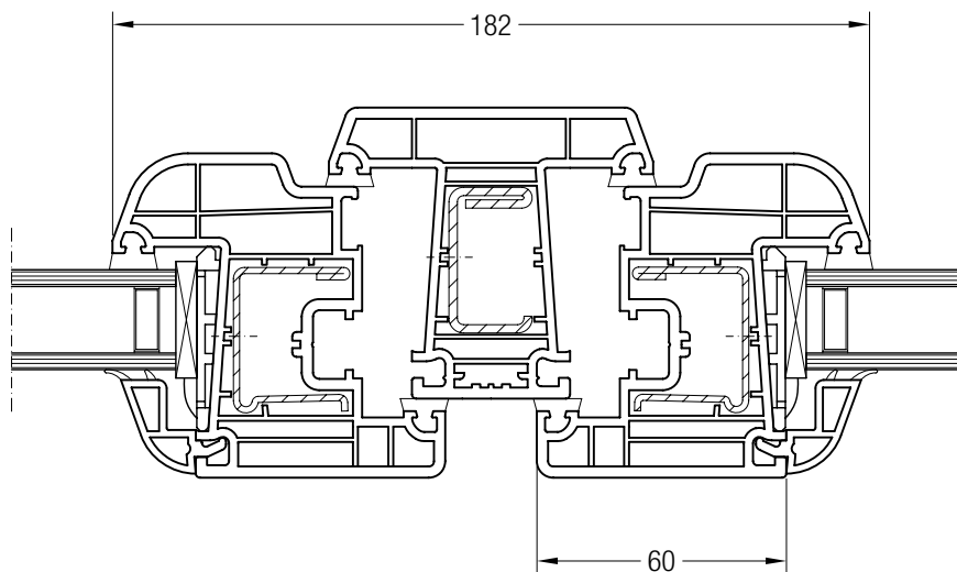
Pfosten 78 ED70 mit Flügel 60 rund ED70, 1550460
