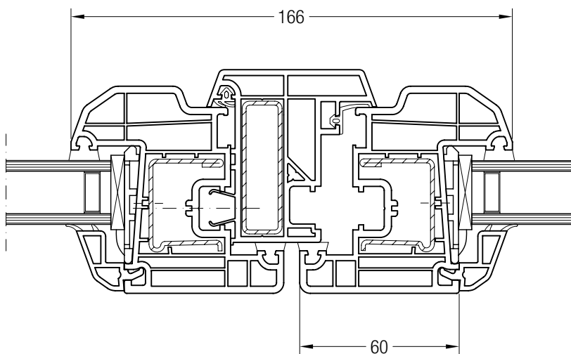
Statik-Blindpfosten Bautiefe 70 mit Flügel A 60 ED70, 1550051
