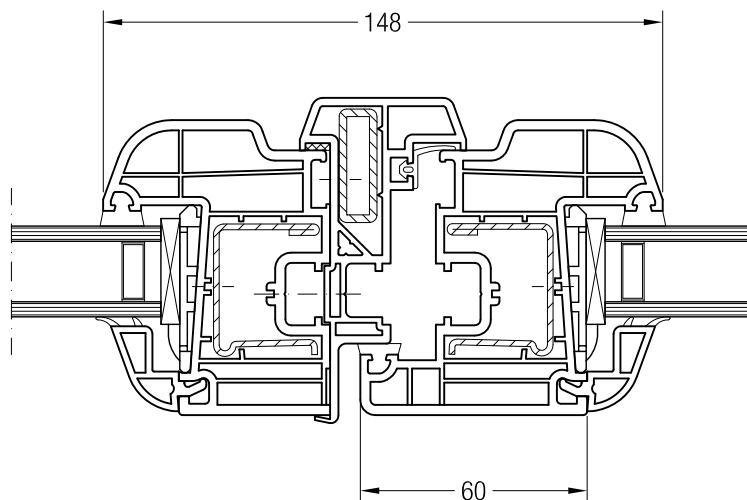
Stulpprofil Bautiefe 70 mit Flügel 60 rund ED70, 1550460
