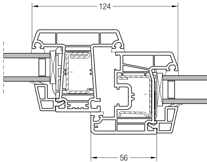
Pfosten 78 ED70 mit Flügel Z 54 ED70, 1550810
