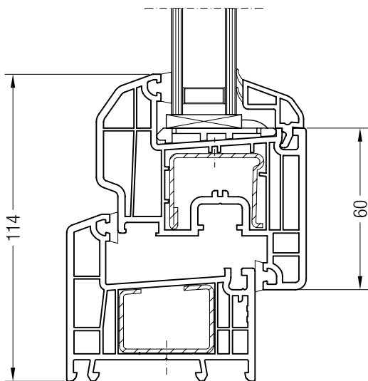
Blendrahmen 62 ED70 mit Flügel A 60 ED70, 1550051
