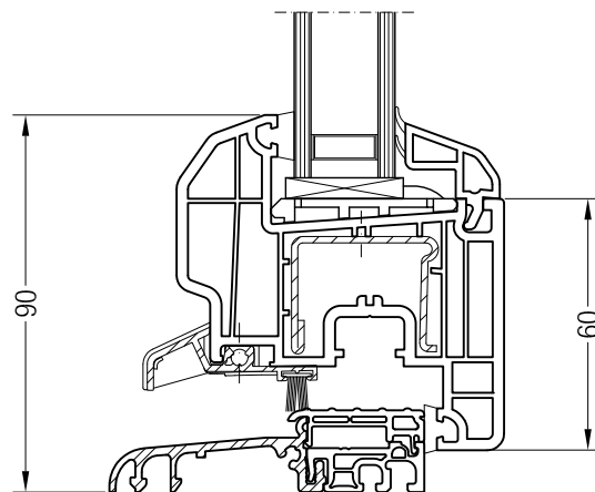
Bodenschwelle 20 Bautiefe 70 mit Flügel A 60 ED70, 1550051
