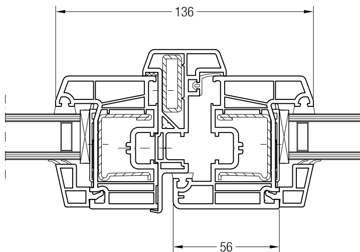
Stulpprofil Bautiefe 70 mit Flügel Z 54 ED70, 1550810
