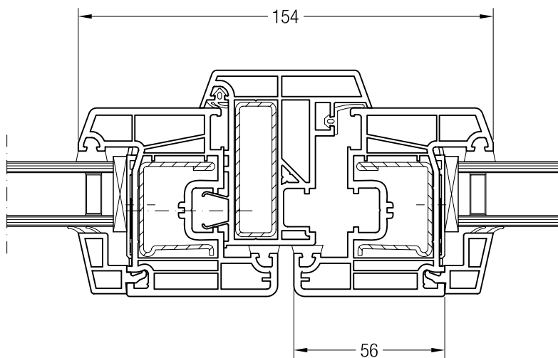
Statik-Blindpfosten Bautiefe 70 mit Flügel Z 54 ED70, 1550810
