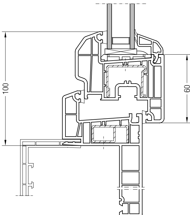
Altbau-Blendrahmen 37 bzw. 60 ED70 mit Flügel A 60 ED70, 1550051
