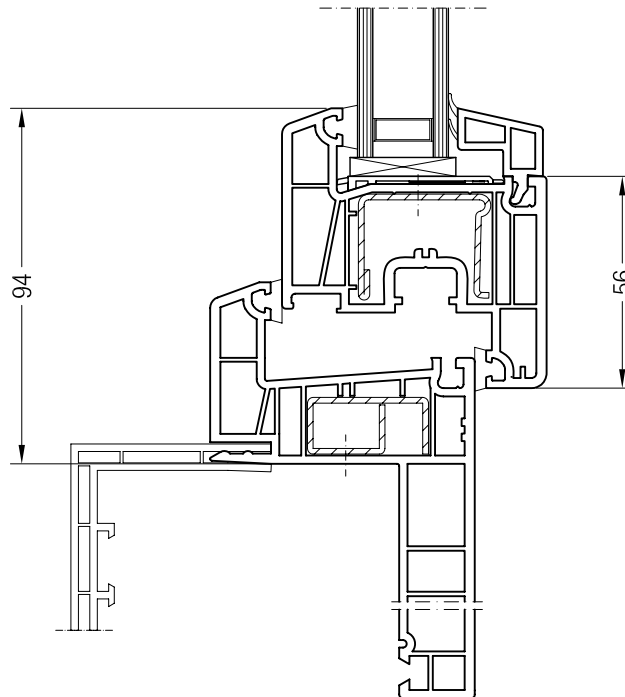
Altbau-Blendrahmen 37 bzw. 60 ED70 mit Flügel Z 54 ED70, 1550810
