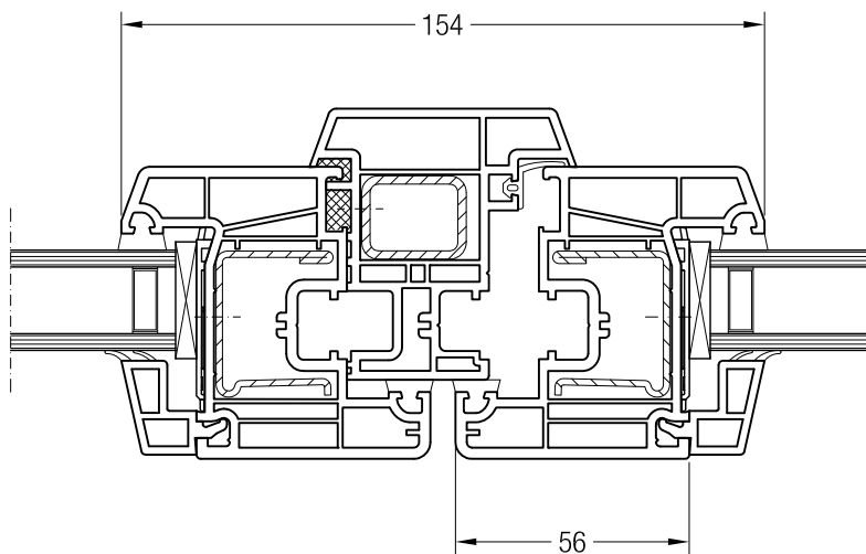
Blindpfosten Nr. 1 Bautiefe 70 mit Flügel Z 54 ED70, 1550810
