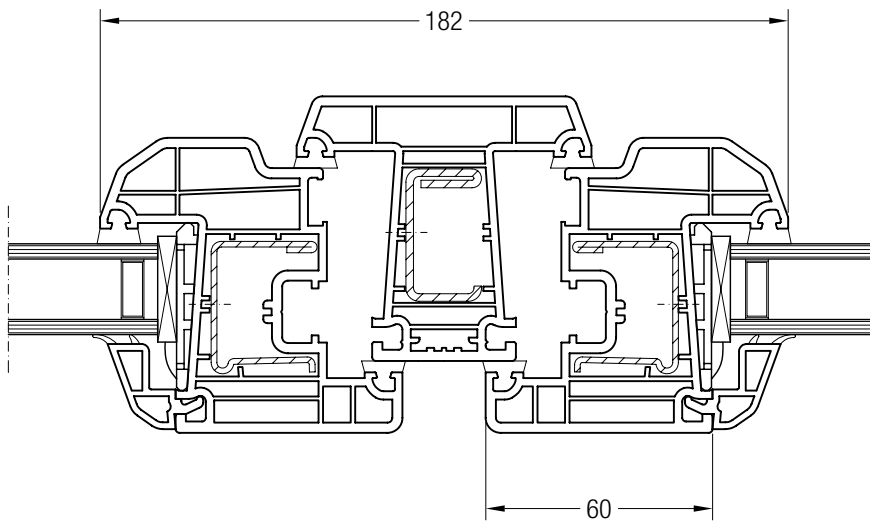
Pfosten 78 ED70 mit Flügel A 60 ED70, 1550051
