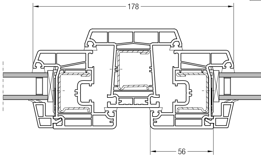
Pfosten 86 ED70 mit Flügel Z 54 ED70, 1550810
