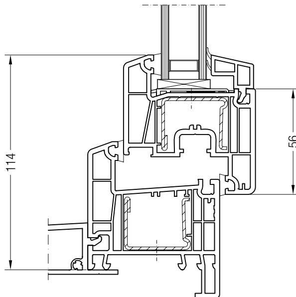
Basis-Blendrahmen 68 ED70 mit Flügel Z 54 ED70, 1550810
