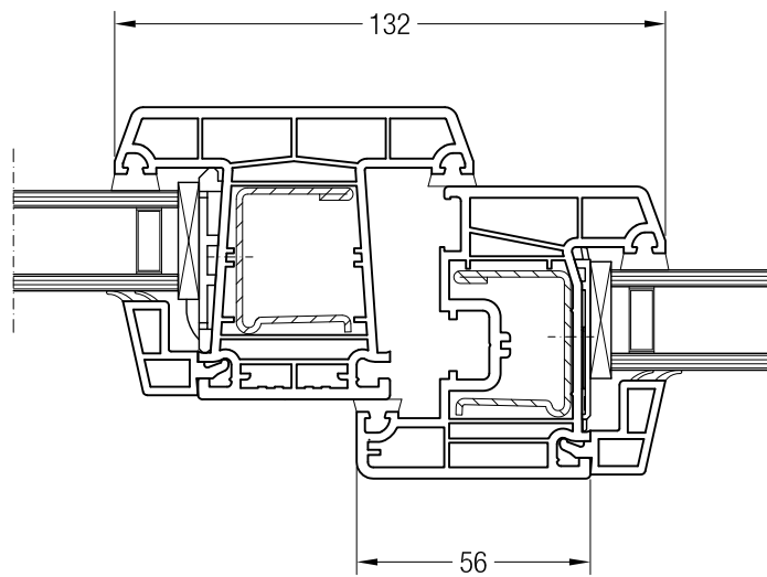
Pfosten 86 ED70 mit Flügel Z 54 ED70, 1550810
