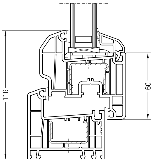
Blendrahmen 64 ED70 mit Flügel A 60 ED70, 1550051
