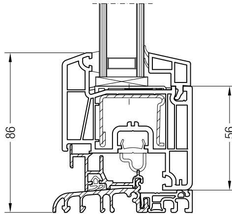
Bodenschwelle 20 Bautiefe 70 mit Flügel Z 54 ED70, 1550810
