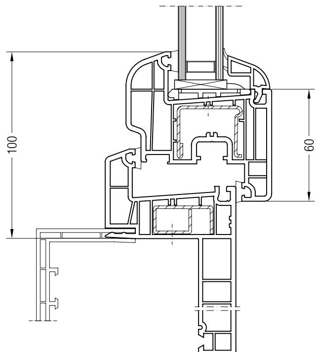
Altbau-Blendrahmen 37 ED70 mit Flügel 60 rund ED70, 1550460
