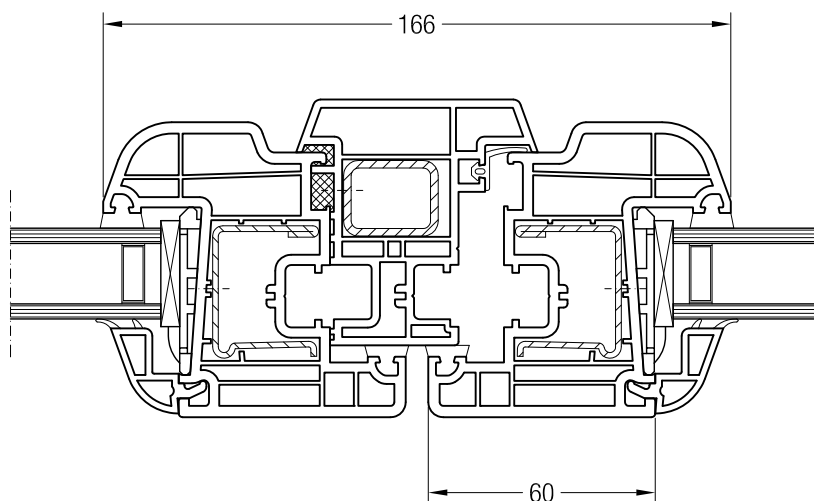
Blindpfosten Nr. 1 Bautiefe 70 mit Flügel 60 rund ED70, 1550460
