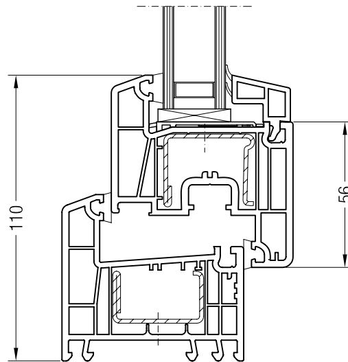
Blendrahmen 64 ED70 mit Flügel Z 54 ED70, 1550810
