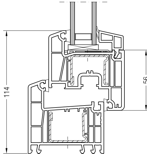
Blendrahmen 68 ED70 mit Flügel Z 54 ED70, 1550810
