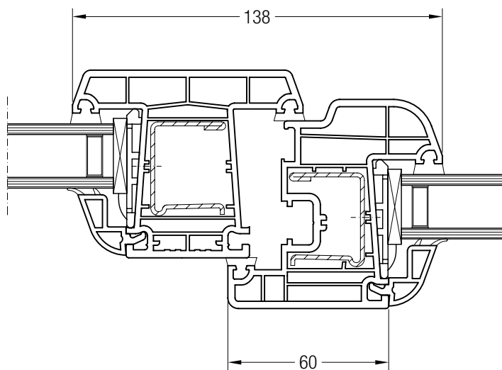
Pfosten 86 ED70 mit Flügel 60 rund ED70, 1550460
