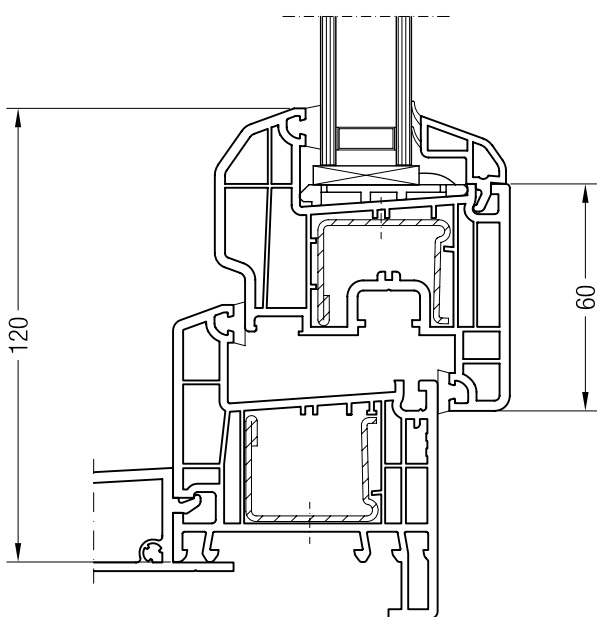
Basis-Blendrahmen 68 ED70 mit Flügel A 60 ED70, 1550051
