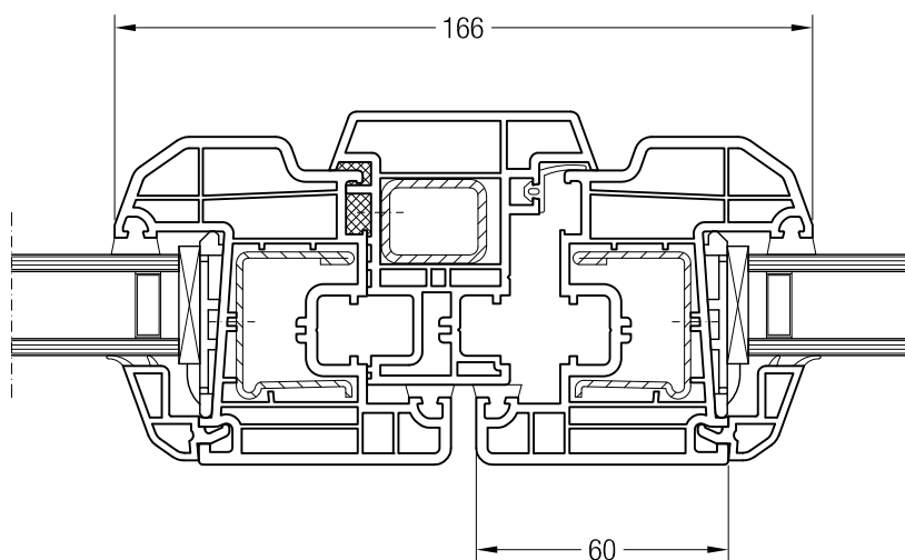
Blindpfosten Nr. 1 Bautiefe 70 mit Flügel A 60 ED70, 1550051
