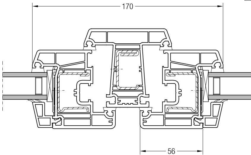
Pfosten 78 ED70 mit Flügel Z 54 ED70, 1550810
