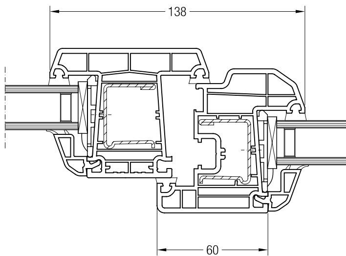
Pfosten 86 ED70 mit Flügel A 60 ED70, 1550051
