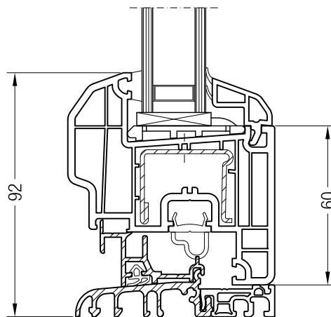
Bodenschwelle 20 Bautiefe 70 mit Flügel A 60 ED70, 1550051
