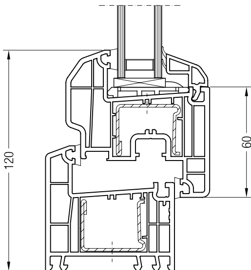
Blendrahmen 68 ED70 mit Flügel A 60 ED70, 1550051
