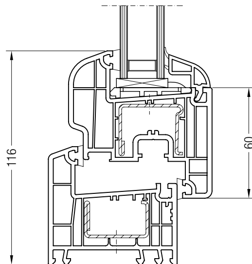
Blendrahmen 64 ED70 mit Flügel 60 rund ED70, 1550460
