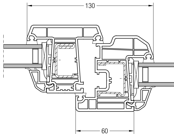
Pfosten 78 ED70 mit Flügel A 60 ED70, 1550051
