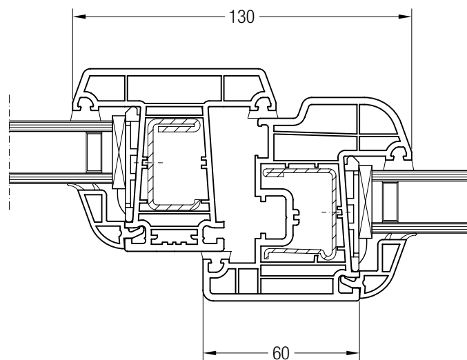
Pfosten 78 ED70 mit Flügel 60 rund ED70, 1550460
