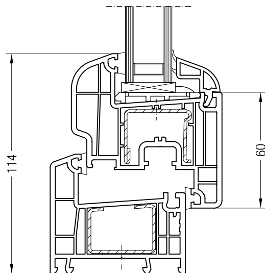
Blendrahmen 62 ED70 mit Flügel 60 rund ED70, 1550460
