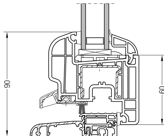
Bodenschwelle 20 Bautiefe 70 mit Flügel 60 rund ED70, 1550460
