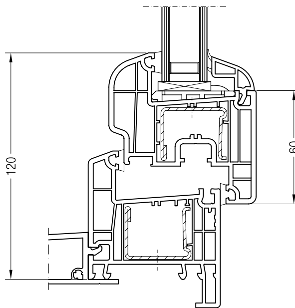
Basis-Blendrahmen 68 ED70 mit Flügel 60 rund ED70, 1550460
