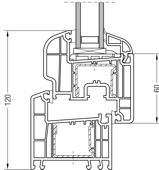
Blendrahmen 68 ED70 mit Flügel 60 rund ED70, 1550460
