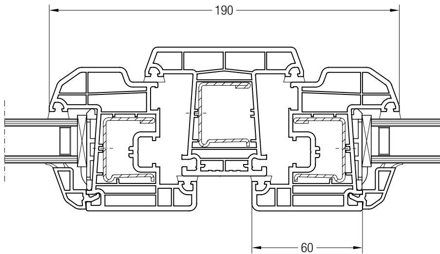
Pfosten 86 ED70 mit Flügel A 60 ED70, 1550051
